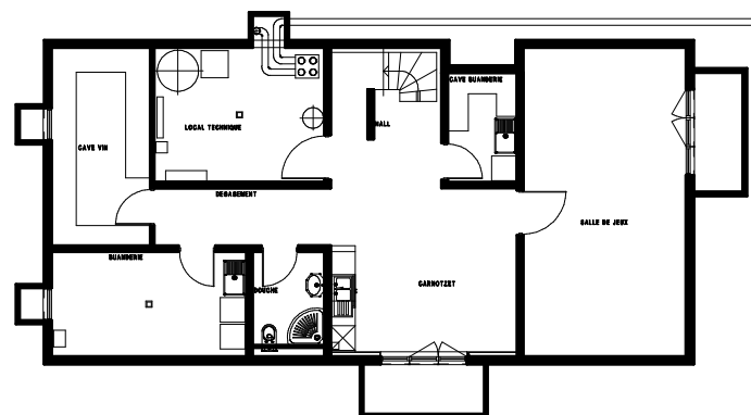
SOUS-SOL 1/200
