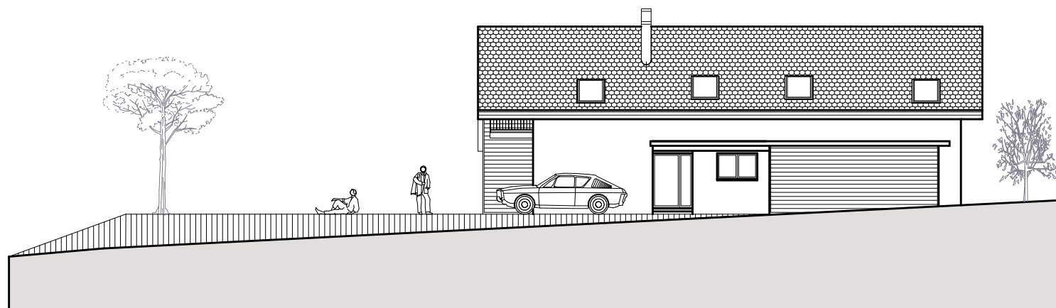
ELEVATION NORD 1/200
